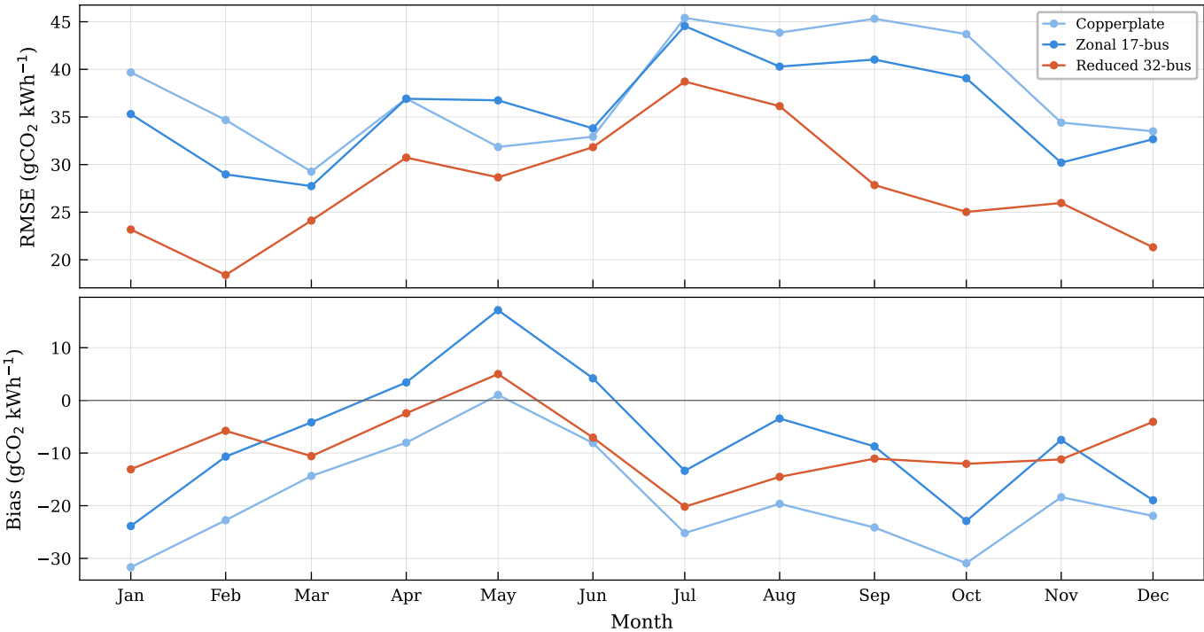
Monthly error metrics vs NESO actual — 2023
